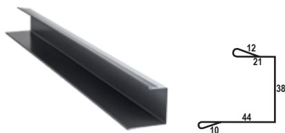
OBR - 10 Profil zamykający do wiatrownicy OBR-08
