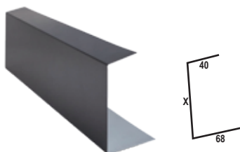
OBR - 04 Pas podrynnowy, bez podęcia
