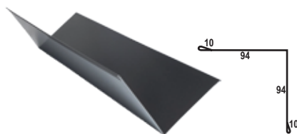
OBR - 14 Narożnik wewnętrzny
