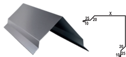
OBR - 15 Narożnik zewn. maskujący
