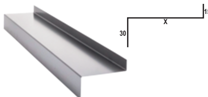
OBR - 20 Listwa startowa
