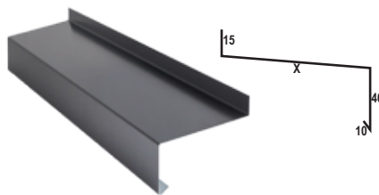
OBR - 17 Okapnik podwalinowy 2
