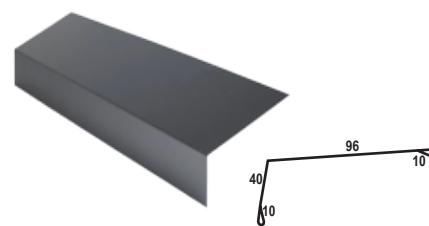
OBR - 06 Maskownica okapu
