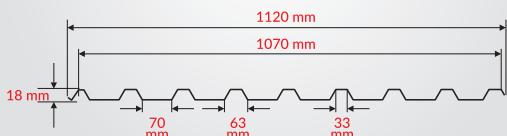
BLACHA TRAPEZOWA T-18 EKO
