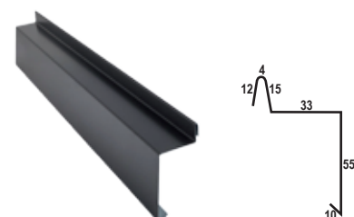
OBR - 21 Okapnik krótki na listwę startową
