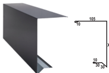
OBR - 08 Wiatrownica do montażu z profilem zamykającym
