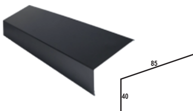
OBR - 11 Maskownica kalenicy
