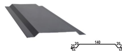
OBR - 12 Maskownica połączeń płyt
