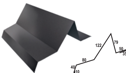
OBR - 05 Maskownica okapu z zaporą śnieżną
