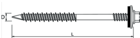
Łączniki do mocowania płyt warstwowych w podłożu betonowym i drewnianym
