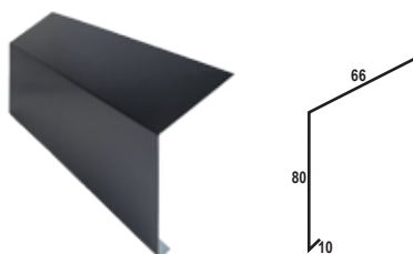
OBR - 07 Pas nadrynnowy
