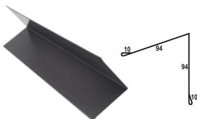
OBR - 19 Narożnik połączenia dach ściana ostry
