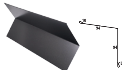
OBR - 18 Narożnik połączenia dach ściana rozwarty
